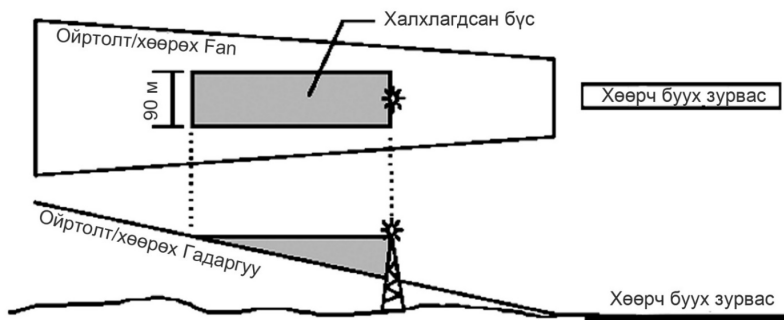
Зураг С.1 - Ойртолт болон хөөрөх гадаргууг халхлах
