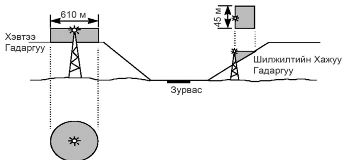
Зураг С.2. - Шилжилтийн болон хэвтээ гадаргууг халхлах
