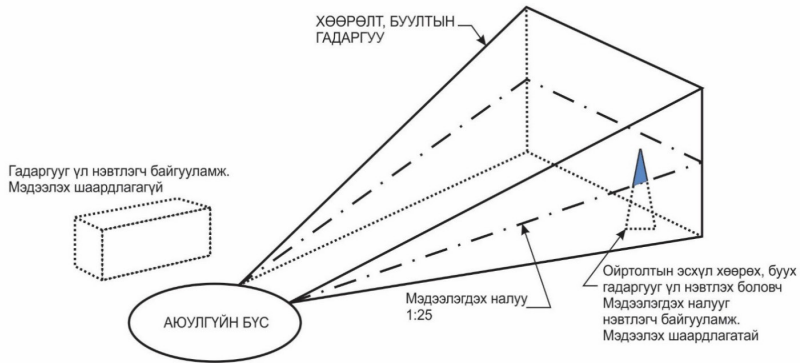
Зураг А.2 - Хелипортын мэдэгдлийн шаардлага
